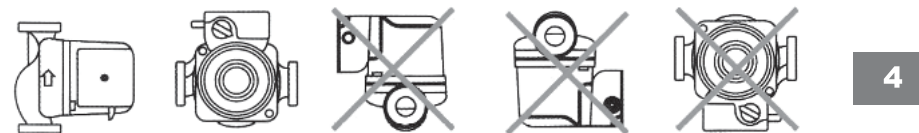
Положение насоса при монтаже
